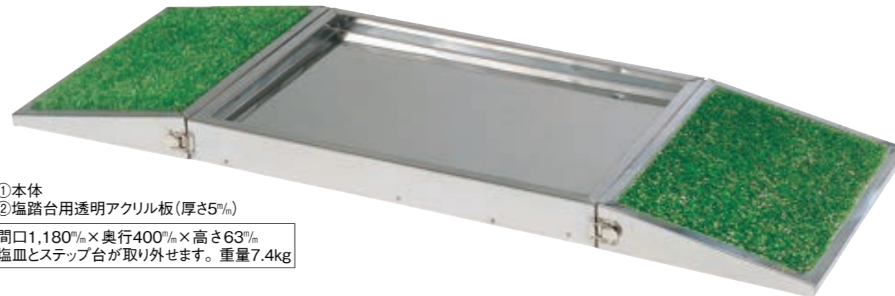
164-1 塩踏台 製品番号 00376
