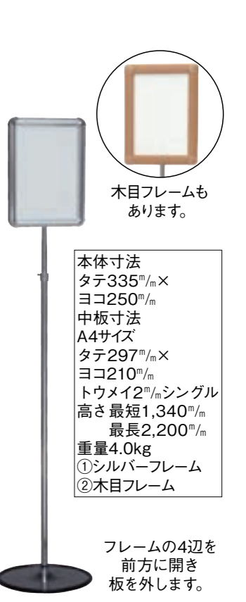
124-8 シルバーフレーム案内板 製品番号 21241
